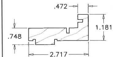
17 ASTRAGAL
