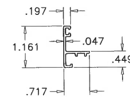
24 ASTRAGAL
